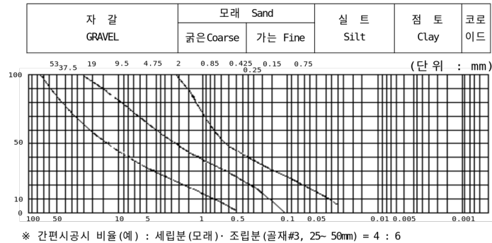
그림 2.2-1 입경분포곡선(grain size accumulation curve)
